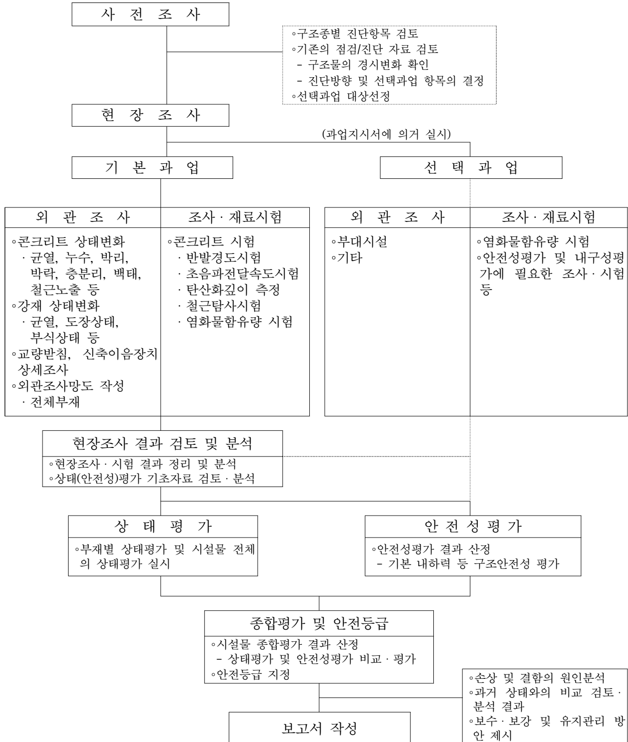
【그림 1.2.1】 정밀안전진단 과업수행 흐름도
