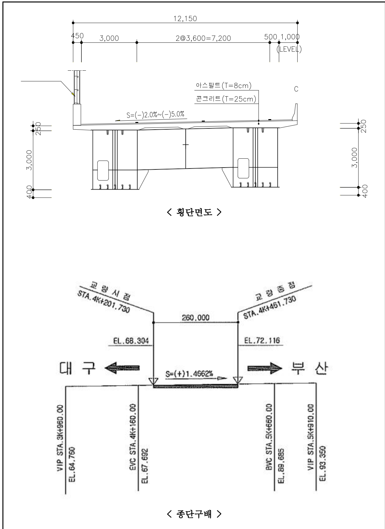
【그림 1.4.6】 시지교(부산) 횡단면도 및 종단구배
