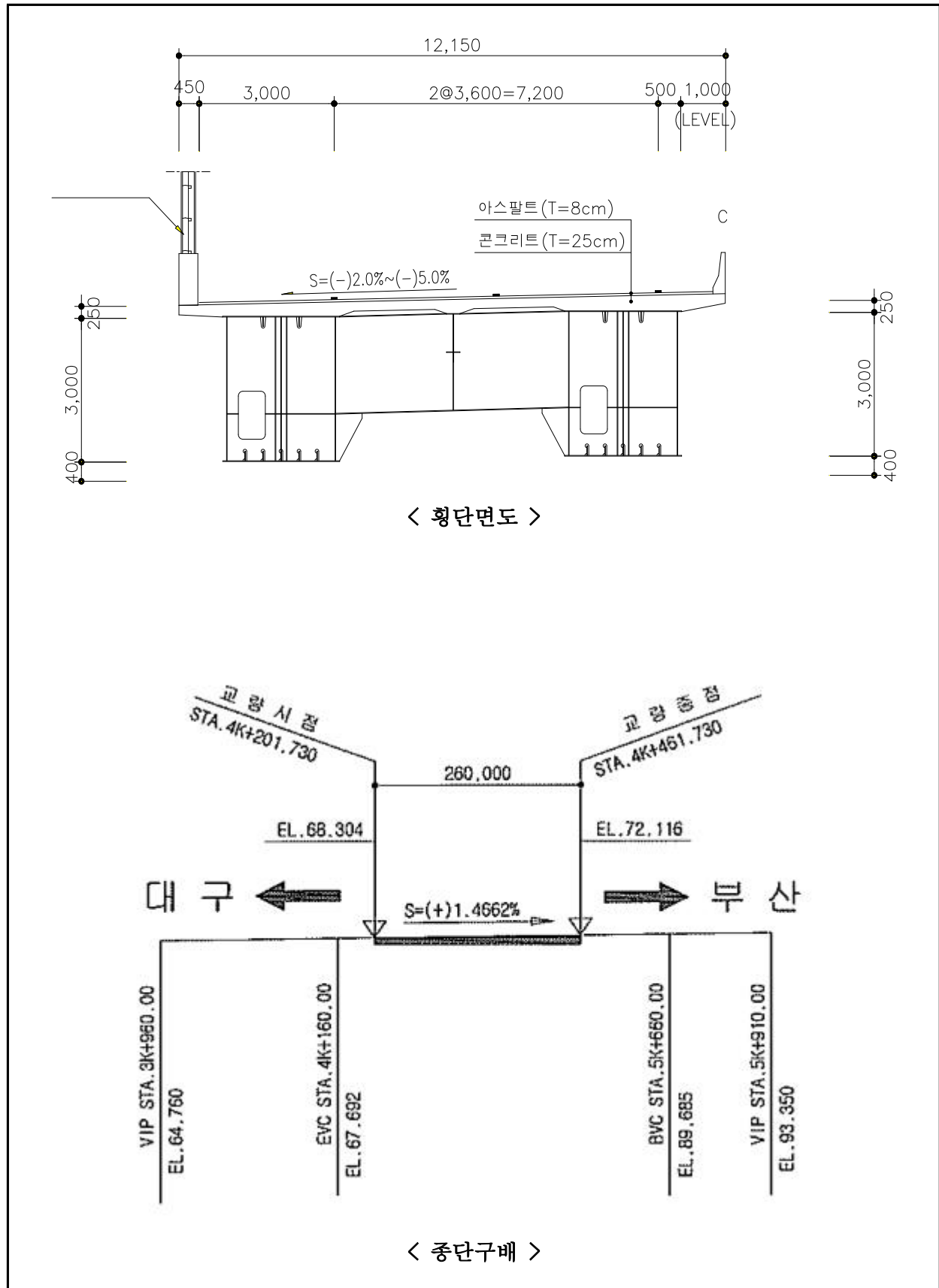
【그림 1.4.2】 시지교(대구) 횡단면도 및 종단구배
