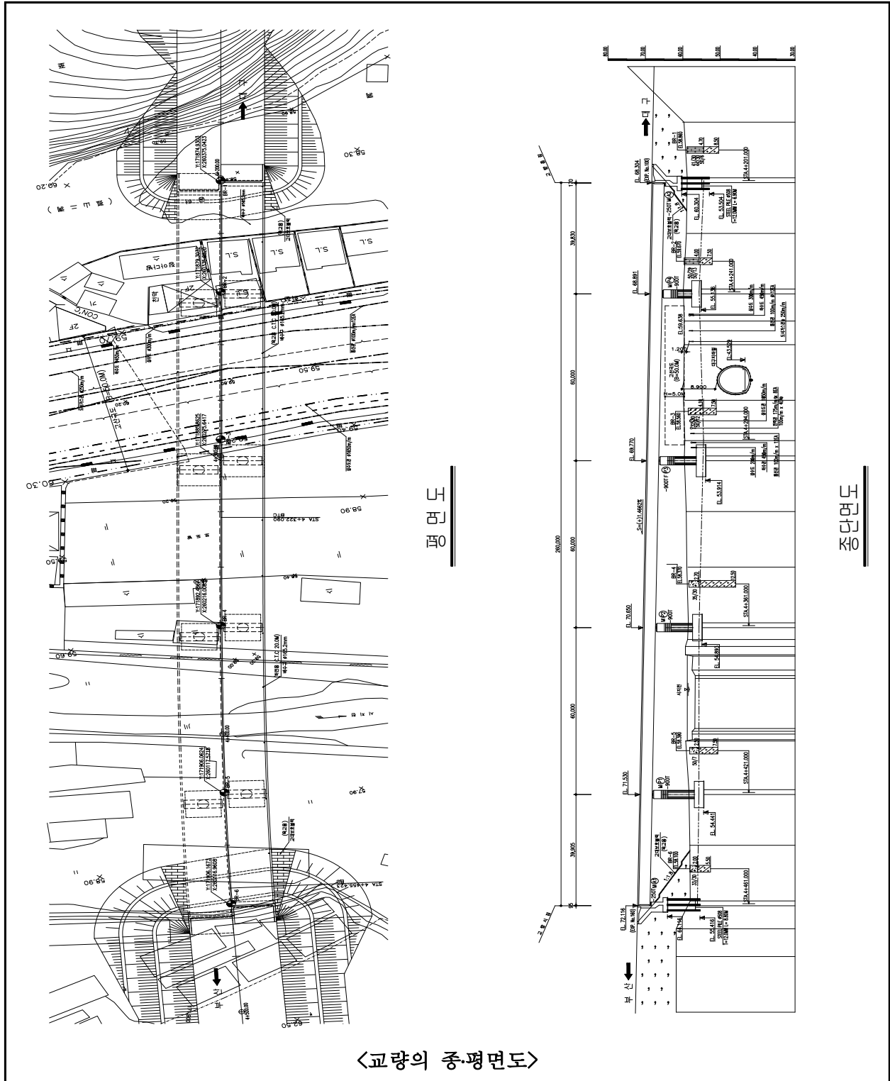
【그림 1.4.1】 시지교(대구) 중·평면도
